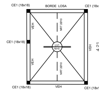
ESTRUCTURA TANQUE RESERVA Esc 1:100
